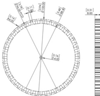
1X 32 Gear 48T Scale 1:1
