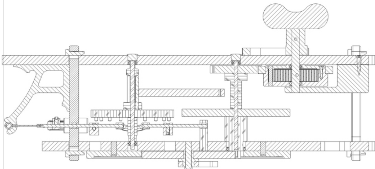
SECTION P-P SCALE 1 : 1
