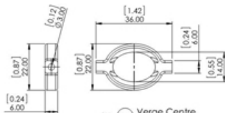
1X (14) Verge Centre Scale 1:1
