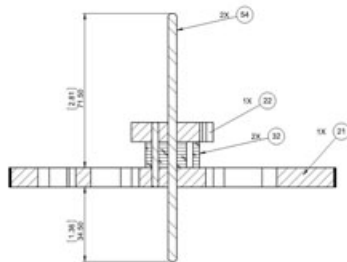
SECTION V-V SCALE 1:1
