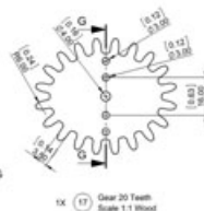
1X 17 Gear 20 Teeth Scale 1:1 Wood
