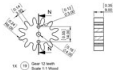
1X 19 Gear 12 teeth Scale 1:1 Wood
